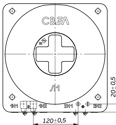
Рис.5-Общий вид трансформатора ТШЛ-СВЭЛ-10-4 (остальное см. Рис.1)
