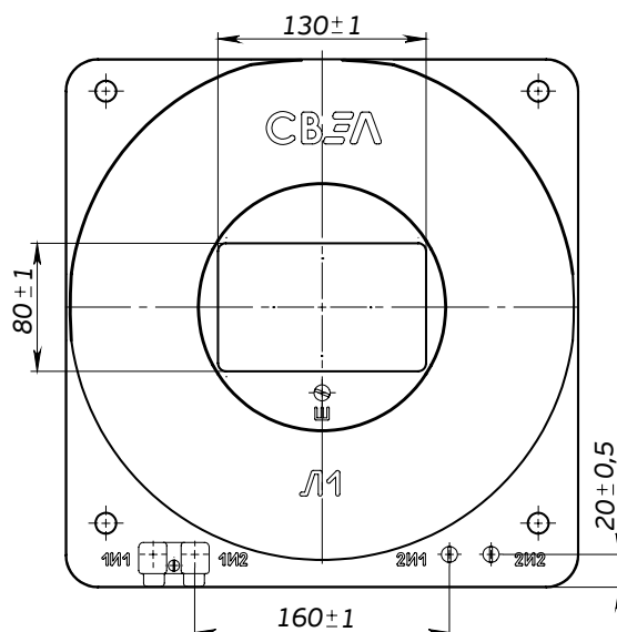
Рис.2-Общий вид трансформатора ТШЛ-СВЭЛ-10-2.2 (остальное см. Рис.1)
